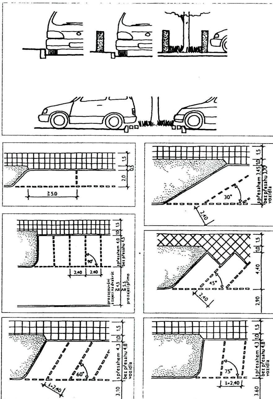
Příklady možného řešení parkovišť pro osobní motorová vozidla. Stromy a travnaté plochy chránějí před bezohlednými motoristy.
