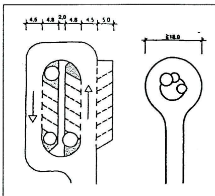
Slepá komunikace s okružním obratištěm, vlevo pro zvýšenou potřebu parkovacích ploch.
