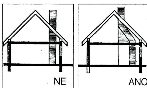
Nevhodné a správné vyústění komínu nad střechou.
