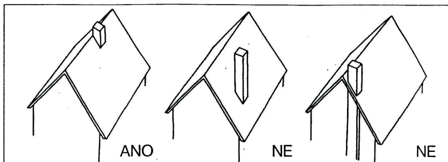
Nevhodné a správné vyústění komínu nad střechou.
