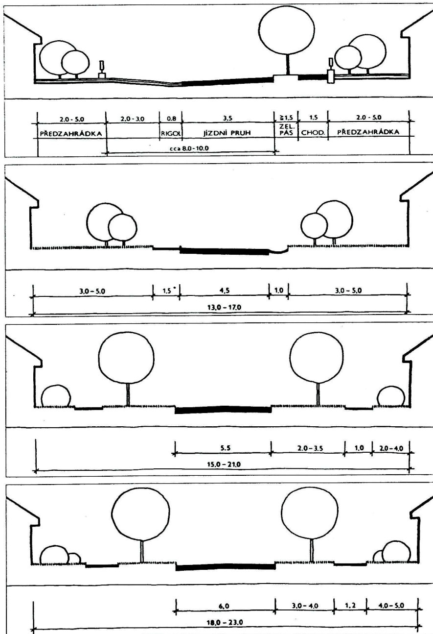
Uliční prostor s vozovkou.
