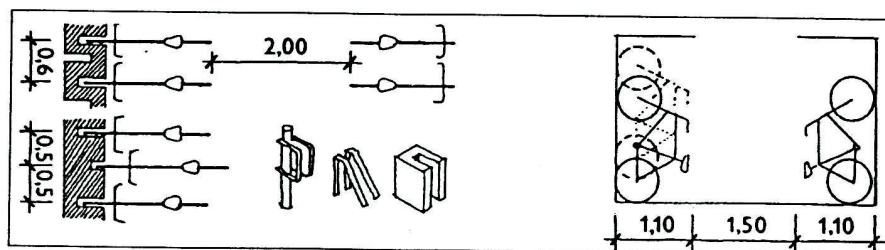
Možné způsoby odstavování bicyklů.
