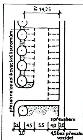
Možné řešení parkování na náběhích a v místech s koncentrací občanského vybavení. Zeleň je chráněna sloupky - pacholíky.
