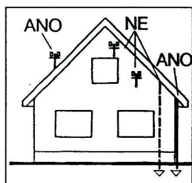
Nevhodné a správné umístění nástřešníků a svodů v průčelí domu.
